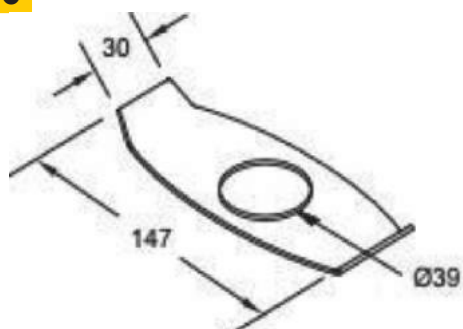
ARRUELA DE ENCOSTO DO EIXO "S" MASTER
