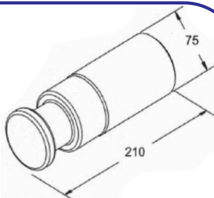
PINO REI CARRETA / SOLDADO COMP 210MM
