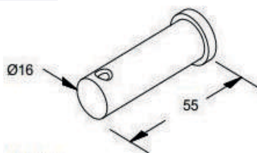
PINO DA FORQUILHA 5/8
