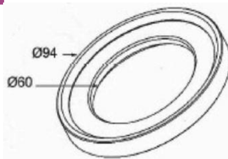
ARRUELA DA BARRA TRAÇÃO COM REBAIXO
