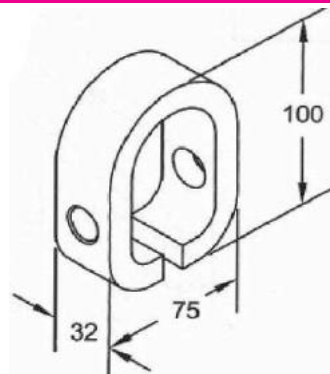
MANCAL DO SUPORTE CENTRAL DA CAR. RANDON PARA PINO 50MM
