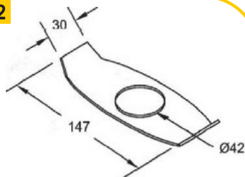
ARRUELA DE ENCOSTO DO EIXO "S" TUBLES
