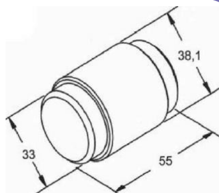
ROLETE PATIM GUERRA MOD. (38,1 X 33 X 55)
