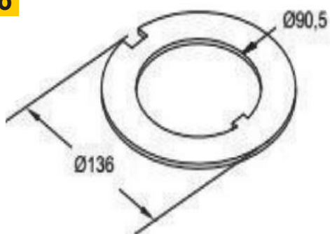
ARRUELA LISA DA CARRETA GUERRA ATÉ 2000 136 X 90,5
