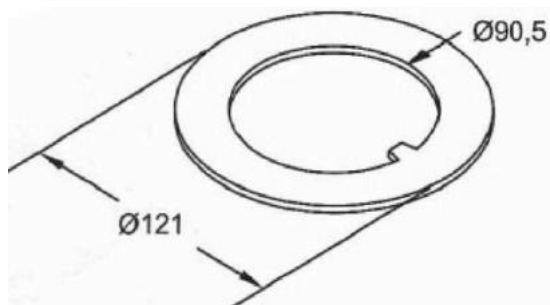
ARRUELA LISA NOMA / IDEROL / KRONE / PASTRE / FACCHINI 121 X 90,5
