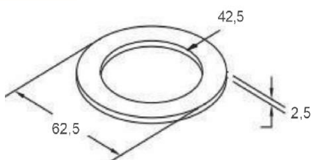
ARRUELA DO EIXO "S" TODOS 62,5 X 42,5 X 2,5MM
