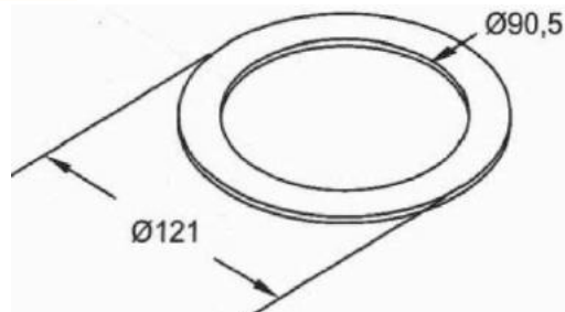
ARRUELA ENCOSTO ROLAMENTO 121 X 90,5 NOMA / IDEROL / KRONE / PASTRE / FACCHINI COM 1,5MM
