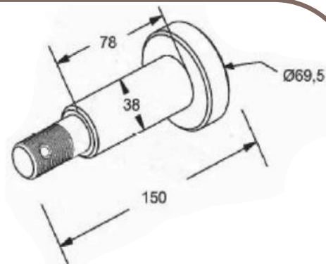
PINO DO TENSOR TRUCK GOYDO (ROSCA 1" 14FPP)
