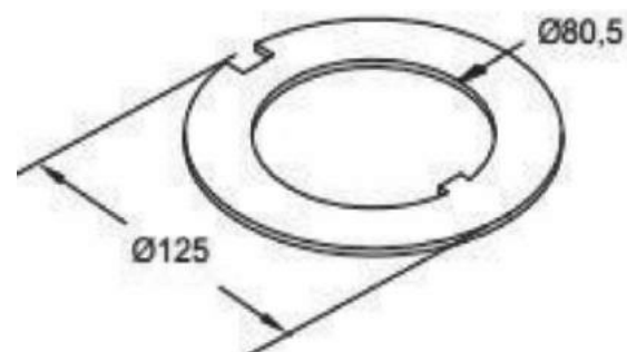
ARRUELA LISA DA CARRETA MOD. 2001 125 X 80,5
