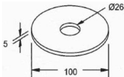
ARRUELA DO PINO CABEÇALHO COD 1230 / 1231 (ROSCA)
