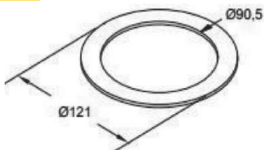
ARRUELA ENCOSTO ROLAMENTO 121 X 90,5 NOMA / IDEROL / KRONE / PASTRE / FACCHINI COM 2MM
