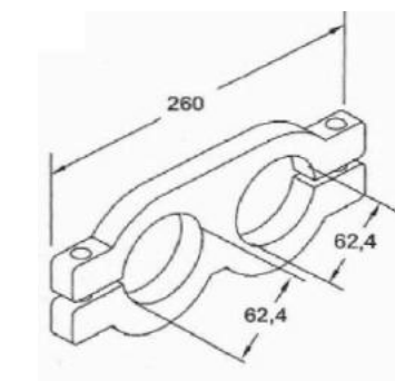
MANCAL DUPLO EXTERNO PINO TENSOR RODOVIÁRIA Ø 62,4MM
