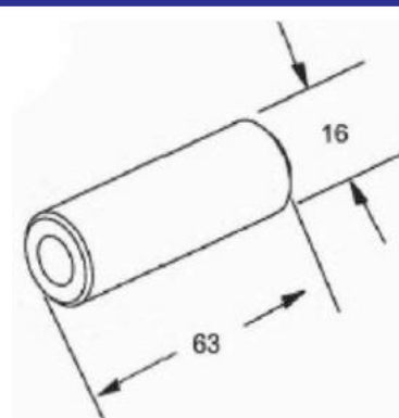
PINO DA BARRA DE TRAVAMENTO QUINTA RODA MAXION
