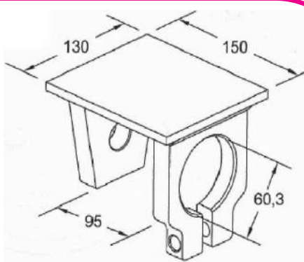
MANCAL RETO DO PINO TENSOR GUERRA Ø60,3MM ABERTURA 95MM
