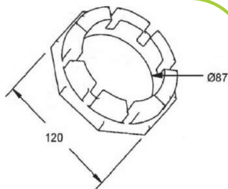
PORCA DO EIXO DA CARRETA FNV
