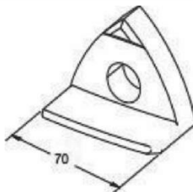
CASTANHA DA RODA CARRETAS / SCANIA MODERNA ABA CURTA
