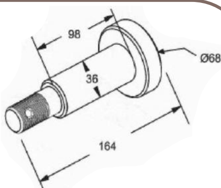
PINO DO TENSOR CANAVIEIRO GALEGO (ROSCA 1" 14FPP)
