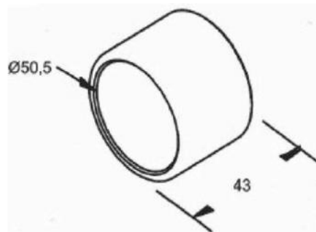
BUCHA DA BARRA TRAÇÃO SEM ABA
