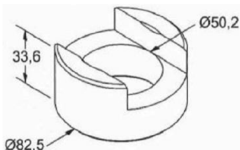
MANCAL EXT. DO PINO DA BALANÇA CARRETA KRONE 82,5 X 50,2 X 33,6
