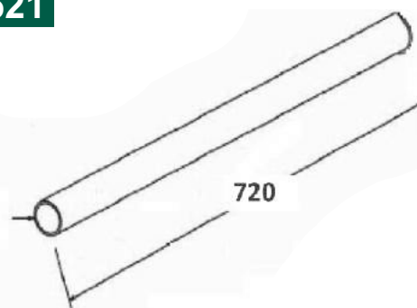
TUBO PARA FIXAÇÃO NO SUPORTE 42 X 2,25 X 720MM
