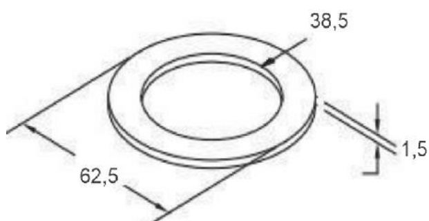
ARRUELA DO EIXO "S" TODOS 62,5 X 38,5 X 1,5MM
