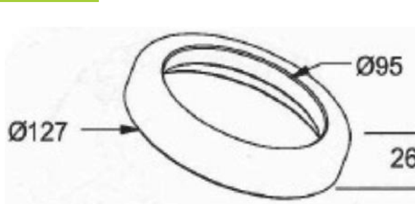
ANEL PISTA DA CARRETA NOMA MODERNA 127 X 95 X 26 COM ENCAIXE
