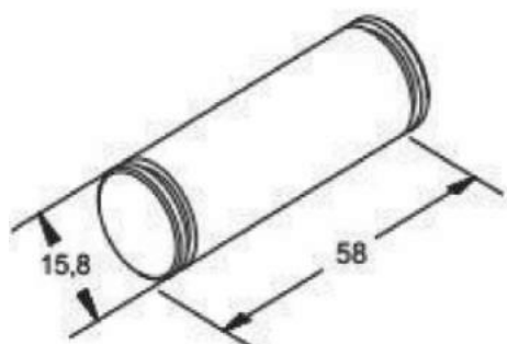
PINO DA ROLDANA TRUCK / CARRETA RODOVIÁRIA (58 X 15,8)
