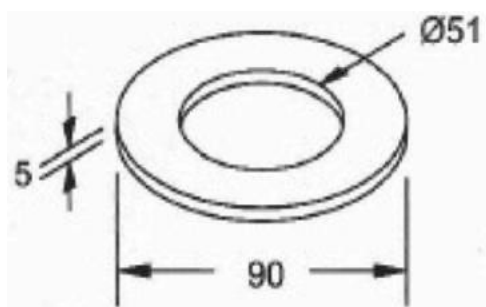
ARRUELA INT. DO PINO CABEÇALHO COD. 1026 / 1027 / 1230 / 1231 (CORPO)
