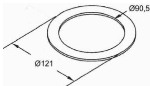
ARRUELA ENCOSTO ROLAMENTO 121 X 90,5 NOMA / IDEROL / KRONE / PASTRE / FACCHINI COM 3MM
