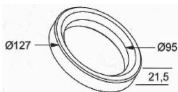
ANEL PISTA RANDOM ANTIGA 127 X 95 X 21,5
