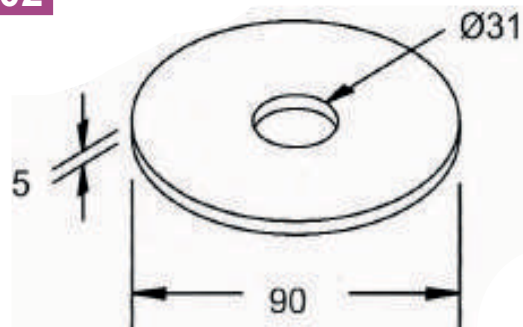
ARRUELA DO PINO CABEÇALHO COD 1026 / 1027 (ROSCA)
