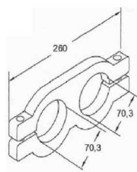
MANCAL DUPLO DO PINO TENSOR RANDON Ø70,3MM
