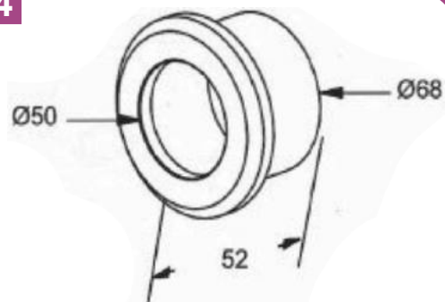
BUCHA DIANTEIRA PONTEIRA CABEÇALHO
