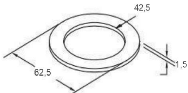
ARRUELA DO EIXO "S" TODOS 62,5 X 42,5 X 1,5MM
