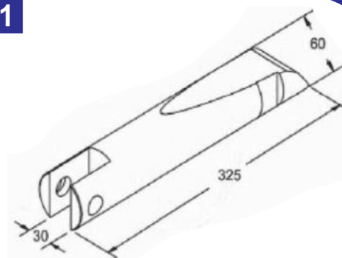
BARRA DE TRAVAMENTO SK38C
