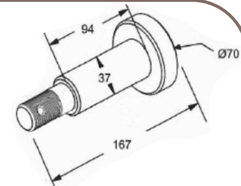
PINO DO TENSOR CARRETA SCHIFFER (ROSCA 1" 14FPP)
