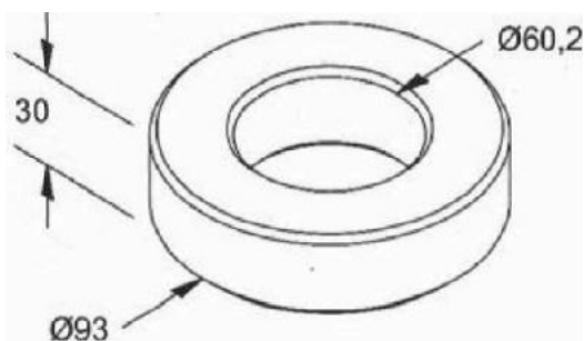
MANCAL INT. DO PINO DA BALANÇA CARRETA KRONE 93 X 60,2 X 30
