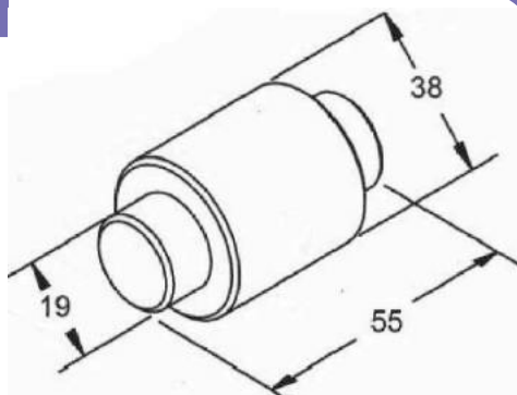
ROLETE SOB MEDIDA 38MM (55 X 38 X 19)
