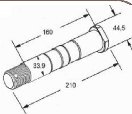
PINO DO TENSOR CARRETA RECRUSUL (ROSCA 1" 1/4 12FPP)
