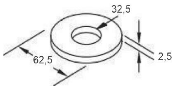
ARRUELA EXTERNA PINO TENSOR FNV 62,5 X 32,5 X 2,5MM
