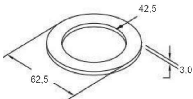
ARRUELA DO EIXO "S" TODOS 62,5 X 42,5 X 3,0MM
