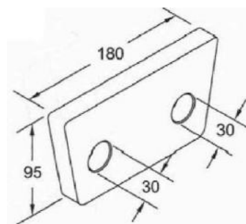
MANCAL DUPLO INT. DO PINO TENSOR RODOVIÁRIA FURO Ø 30MM
