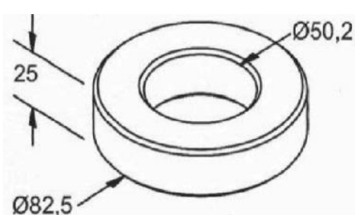
MANCAL INT. DO PINO DA BALANÇA CARRETA KRONE 82,5 X 50,2 X 25
