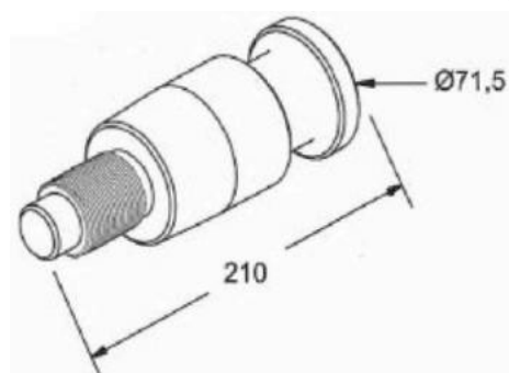
PINO REI DA CARRETA RANDON
