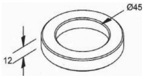
ARRUELA DA PONTEIRA 45MM
