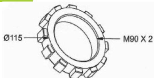
PORCA EIXO CAR. GUERRA / NOMA / IDEROL / FACCHINI / KRONE MOD (M90 X 2)
