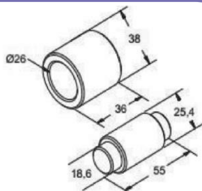
ROLETE DO PATIM COM BUCHA FREIO Á DISCO
