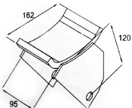
DESLIZANTE CARRETA RODOFORT
