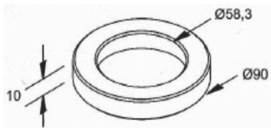
ARRUELA DA BARRA DE TRAÇÃO RANDON 90 X 58,3 X 10MM
