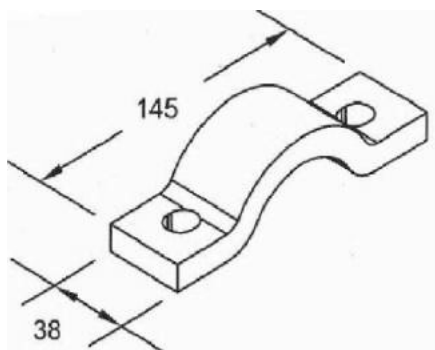
MANCAL GUERRA PARA PINO DA BALANÇA 50MM
