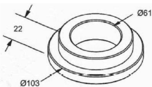
MANCAL INTERNO NOMA 61 X 103 X 22
