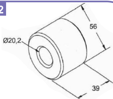
ROLDANA DO PATIM MB (56 X 20,2 X 39)
