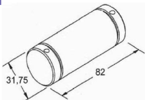
PINO DO PATIM BENDIX ANTIGO (82 X 31,75)
