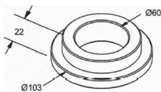
MANCAL INTERNO NOMA 60 X 103 X 22
