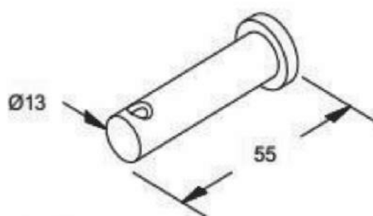
PINO DA FORQUILHA 1/2
