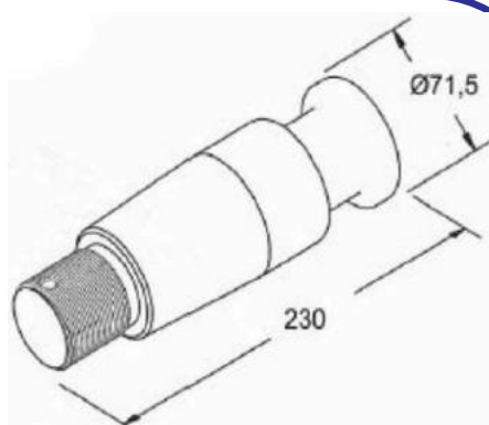
PINO REI DA CARRETA GUERRA
