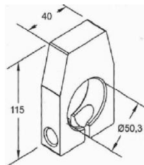
MANCAL EXTERNO TRUCK / CARRETA RODOVIÁRIA Ø 50,3MM
