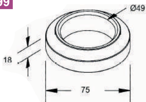
ANEL TRASEIRO DA BARRA TRAÇÃO
