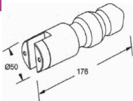
PINO DO ENGATE RANDON MODERNO
