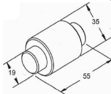
ROLETE SOB MEDIDA 35MM (55 X 35 X 19)
