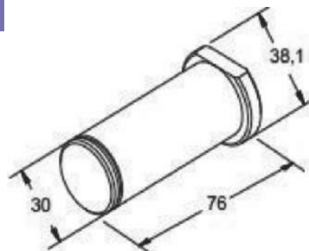
PINO DA FLANGE TRUCK / CARRETA RODOVIÁRIA ATÉ 80 (76 X 38,1 X 30)
