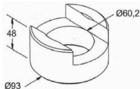
MANCAL EXT. DO PINO DA BALANÇA CARRETA KRONE 93 X 60,2 X 48
